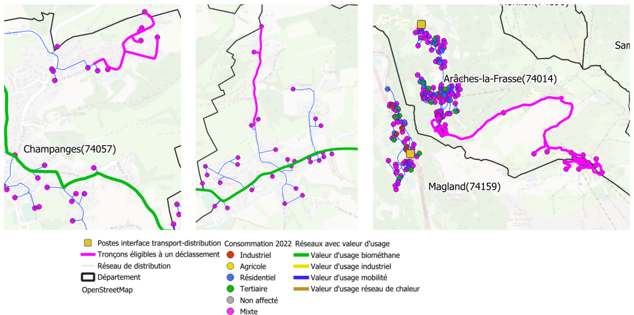
Figure 67 : Focus sur plusieurs parties du réseau éligibles à un déclassement (Haute-Savoie, baisse amplifiée)
