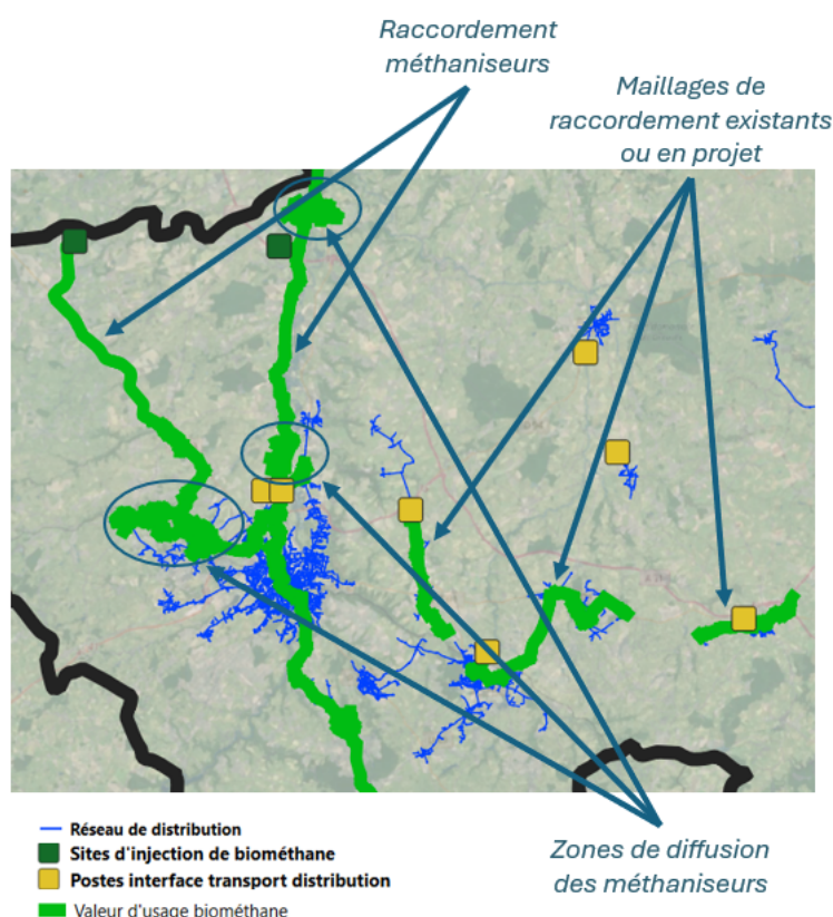
Figure 44 : Détermination des différentes canalisations à valeur d'usage "biométhane"
