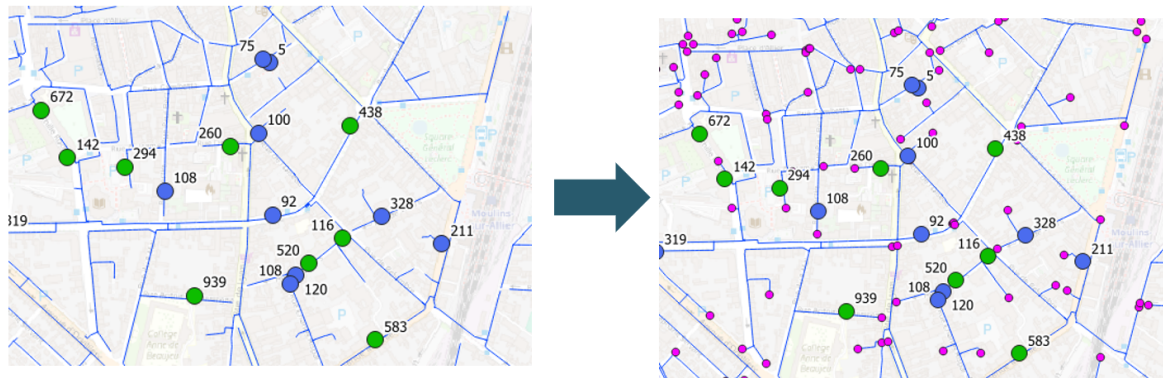
Figure 41 : Exemple sur une IRIS (en rose les consommations affectées aux extrémités du réseau)
