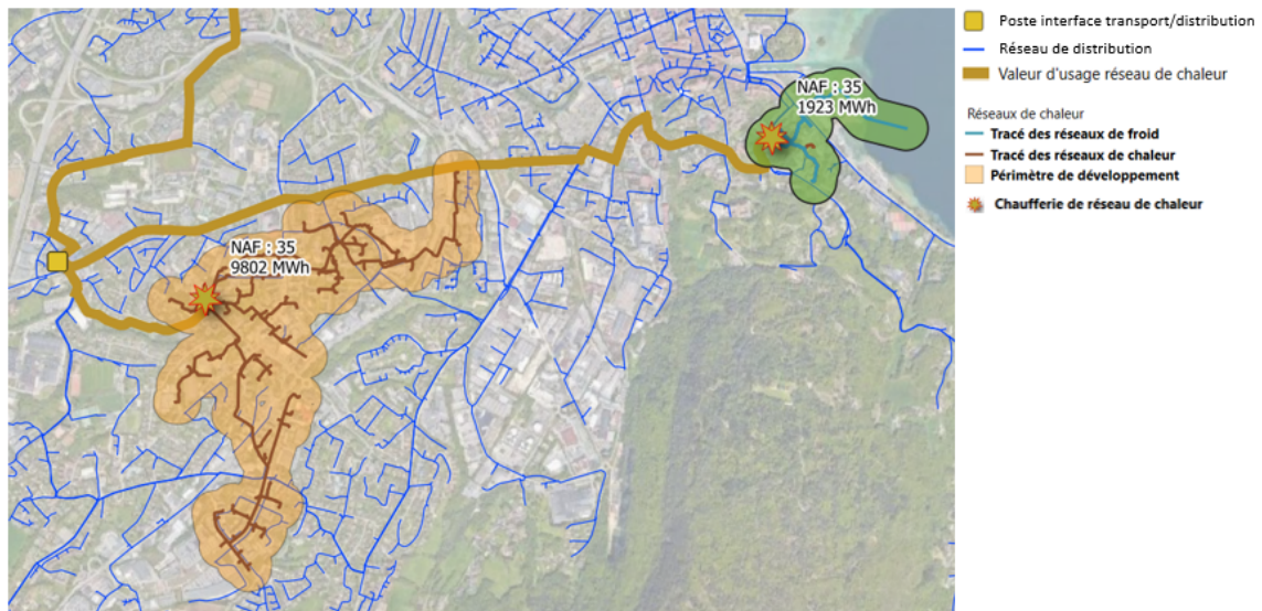
Figure 46 : Sanctuarisation des canalisations de gaz permettant l'appoint/secours d'un réseau de chaleur
