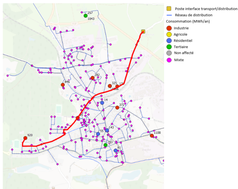
Figure 42 : cheminement du gaz entre un point de consommation et un PITD (en rouge)
