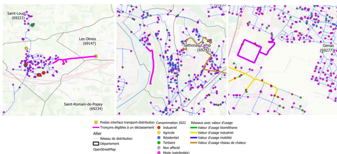
Figure 74 : Focus sur des canalisations éligibles à un déclassement (Rhône, PG24)
