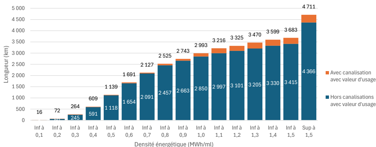
Figure 72 : Longueur de canalisation par densité énergétique - Département du Rhône - Situation 2022
