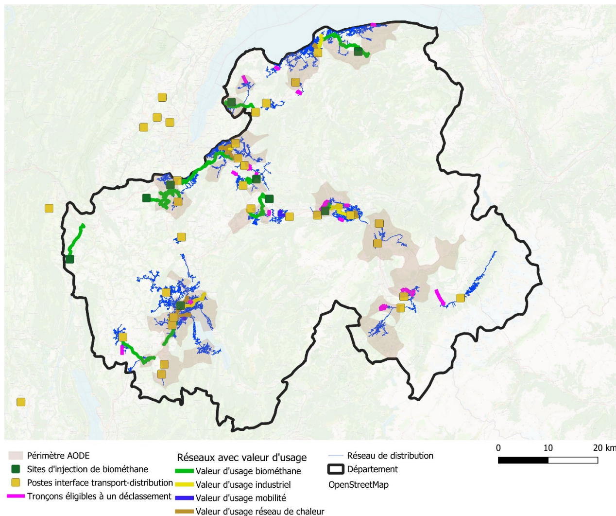
Figure 65 : Localisation des canalisations éligibles à un déclassement (Allier, PG24)
