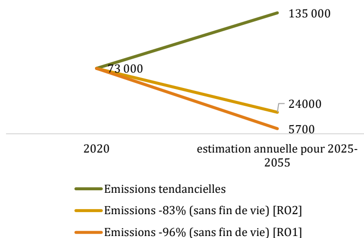
Graphique 2 : Émissions tendancielles et avec restriction universelle dans l'espace économique européen (en tonnes par an)
