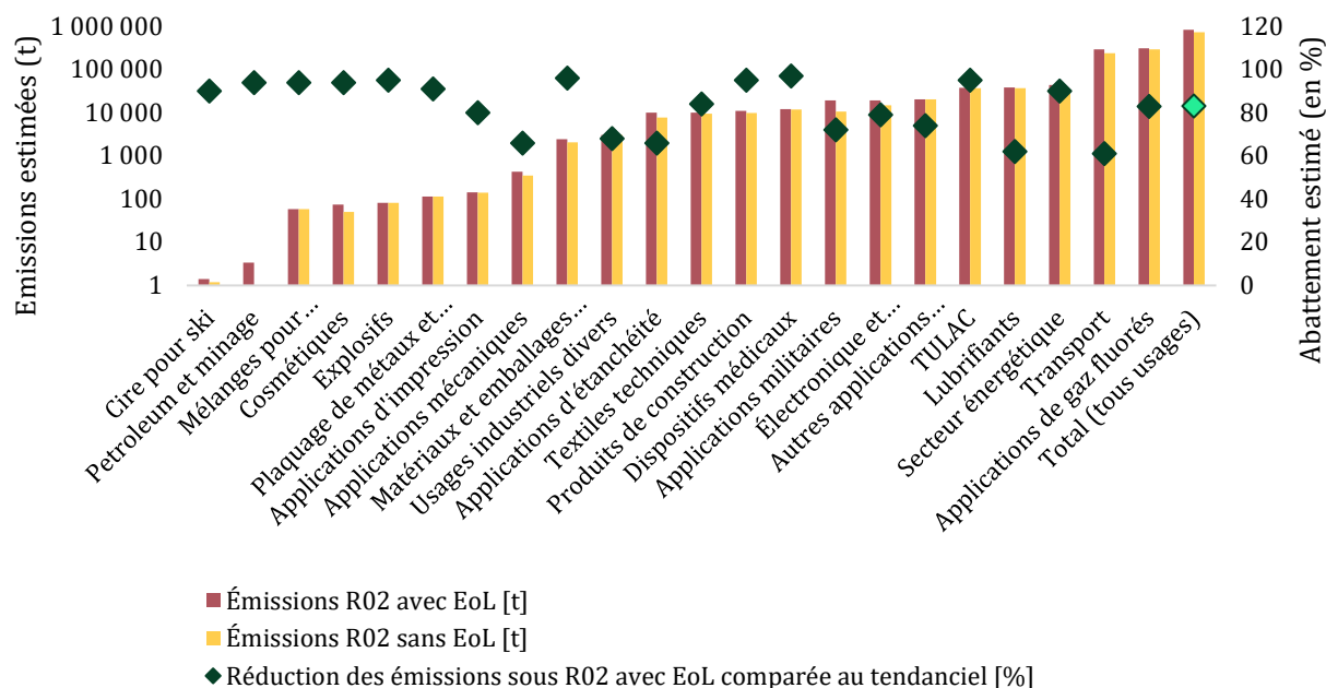
Graphique 4 : Émissions de PFAS estimées sur la période d'évaluation (2025-2055), en tonnes, et abattement estimé par rapport au tendanciel
