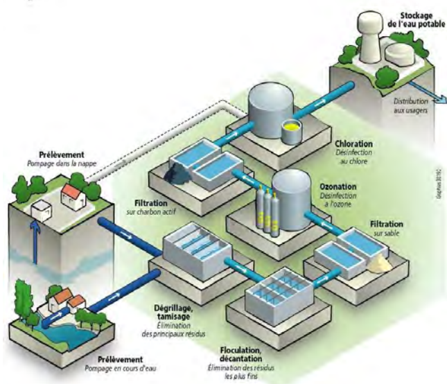
Figure 2 : Les étapes de production de l'eau potable
