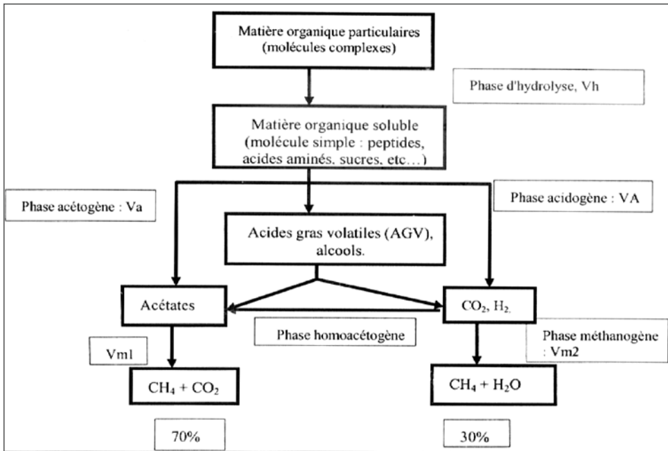
Figure 10 : Étapes biochimiques de la digestion anaérobie [Hédreit, 1993; De La Farge, 1995]
